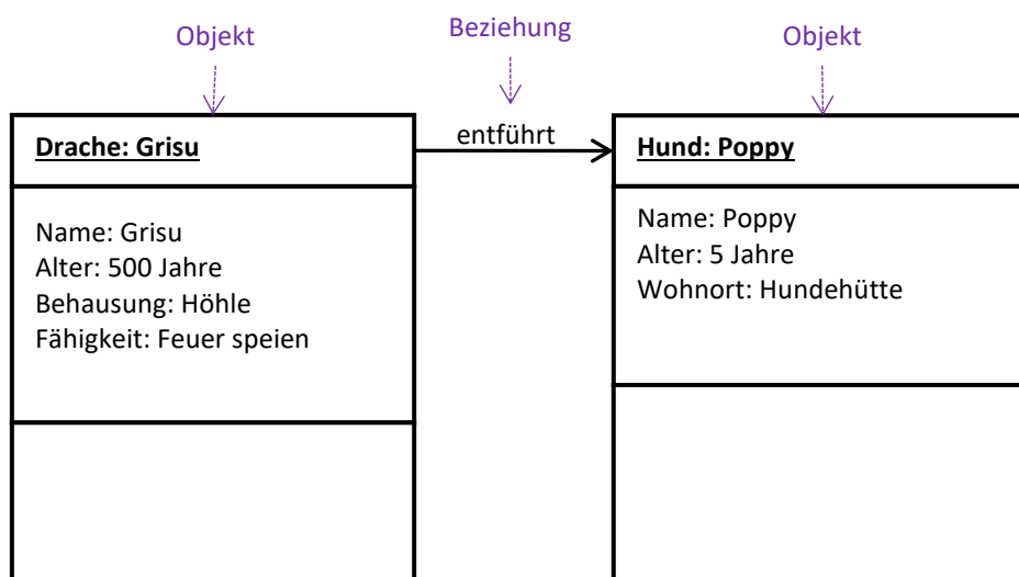
Abbildung 3: Beispiel eines Objektdiagramms
