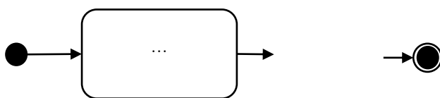
Abbildung 14: Start- und Endzustände im Aktivitätsdiagramm
