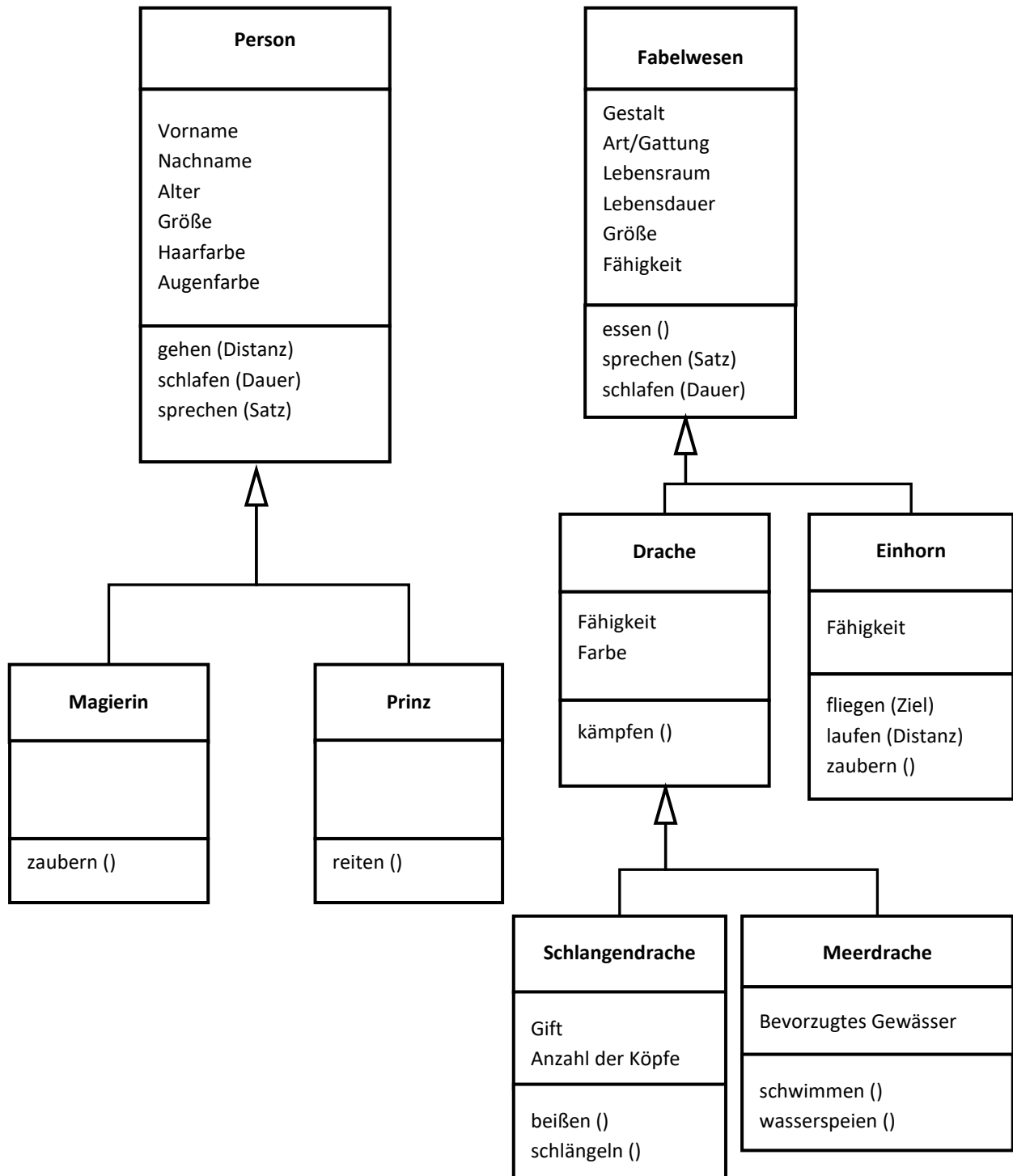
Abbildung 11: Beispiel Klassendiagramm mit Generalisierungen
