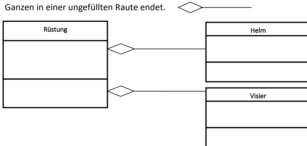
Abbildung 9: Klassendiagramm mit Aggregation
