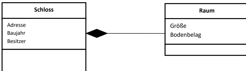
Abbildung 8: Klassendiagramm mit Komposition
