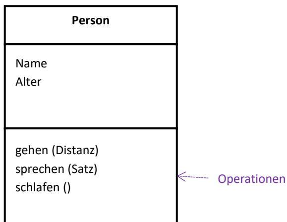
Abbildung 10: Klassendiagramm mit Methoden
