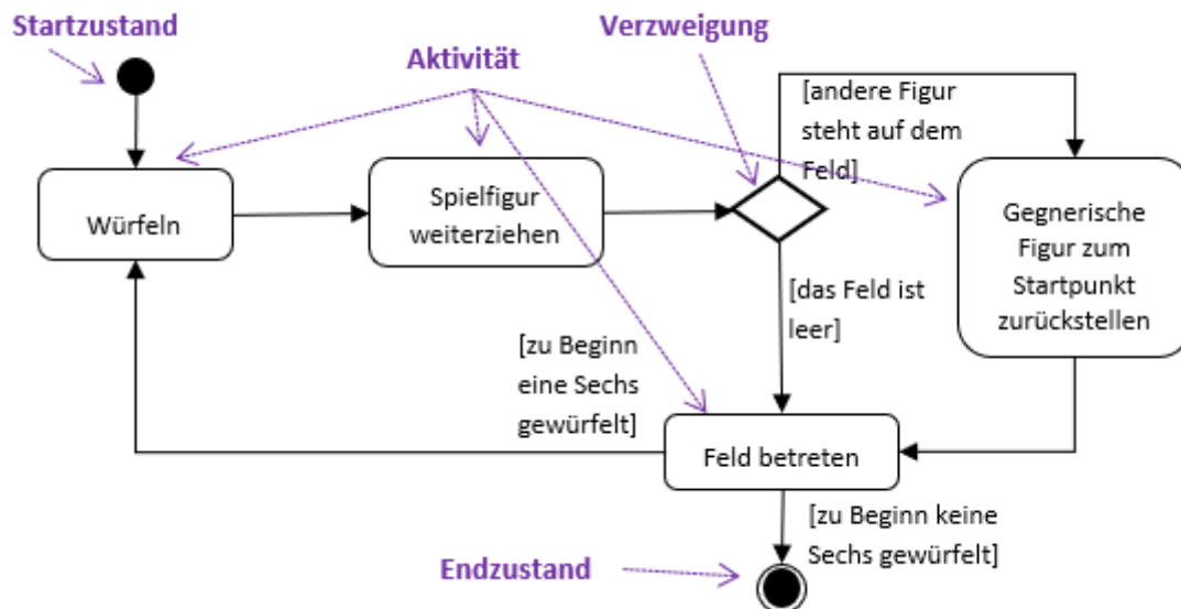
Abbildung 2: Beispiel eines Aktivitätsdiagramms
